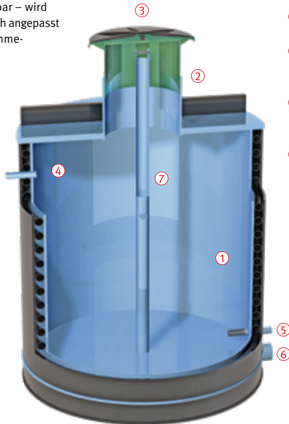
Doppelwandige Bauweise
