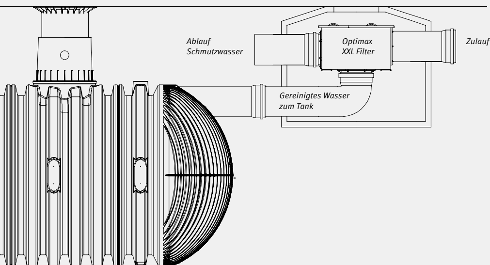
Funktion Filter-Reinigungseinheit
