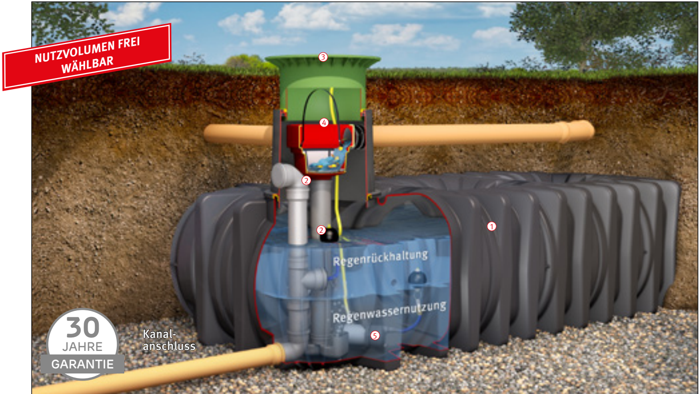
Abb. zeigt Platin XL Retentionszisterne mit Platin XL/XXL Retention Ausbaupaket 2 (Zubehör unten) und Technikpaket Garten-Komfort (Zubehör Seite 42)
