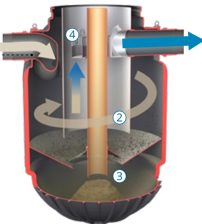
Zweikammersystem
