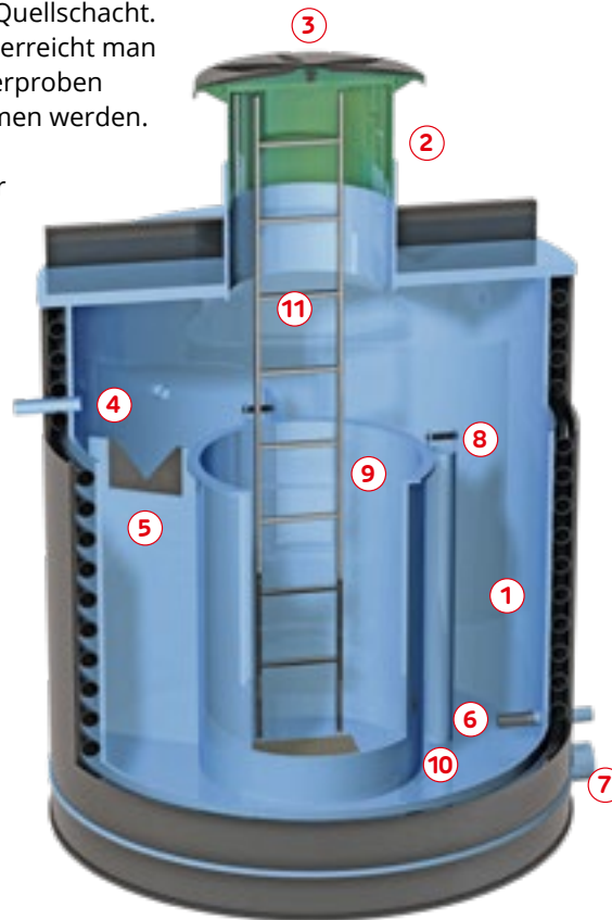
Doppelwandige Bauweise
