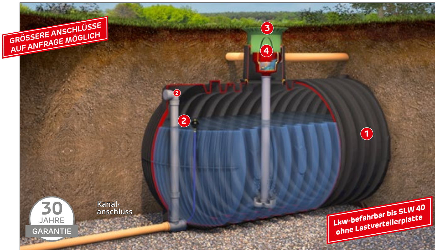
Abb. zeigt Carat XXL Retentionszisterne mit Carat XL/XXL Retention Ausbaupaket 2 (Zubehör Seite 155)
