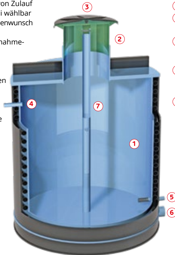
Doppelwandige Bauweise
