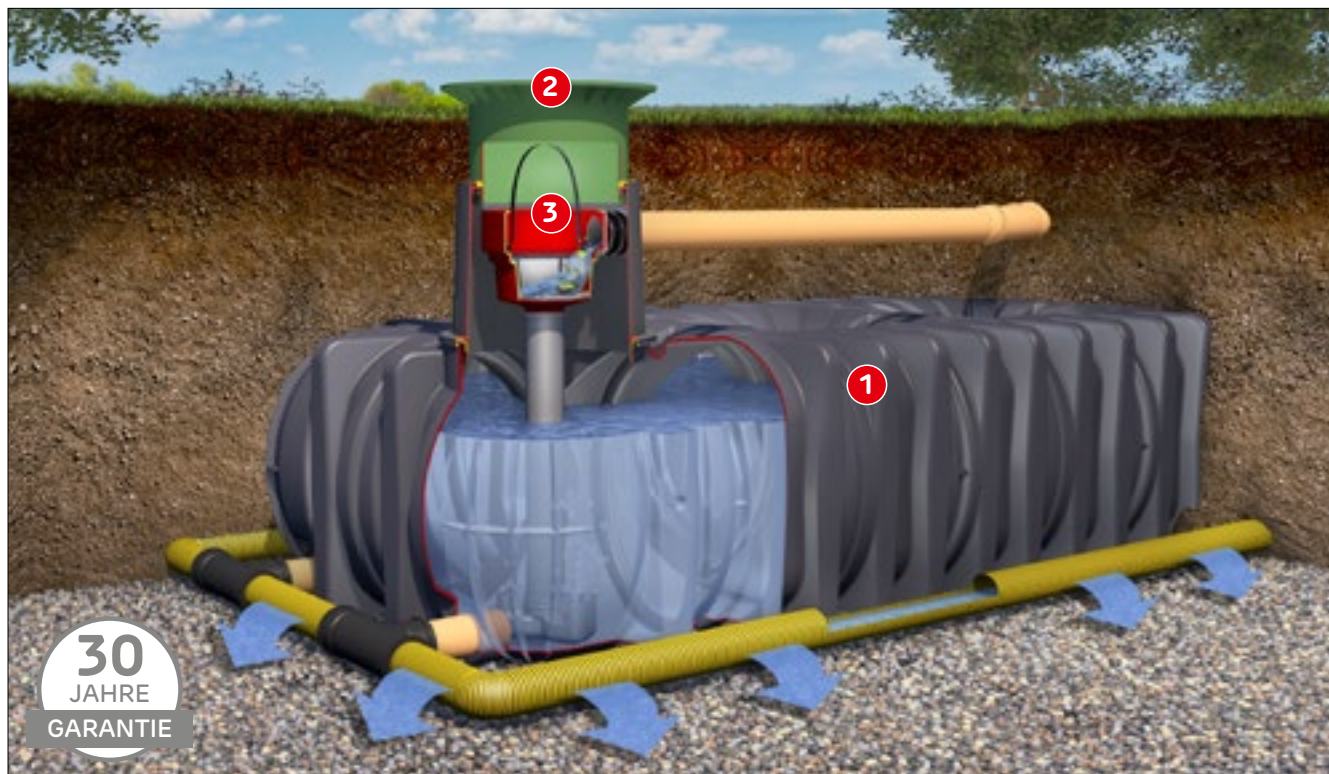
Abbildung zeigt Platin XL Versickerung mit Platin XL Retention/Versickerung Ausbaupaket 2 (siehe Zubehör S. 40)
