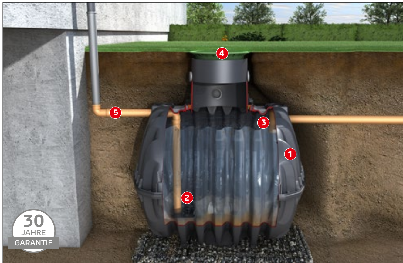
Abbildung zeigt Erdtank Carat M 153 Sedimentationstank mit Lieferumfang und Teleskop-Domschacht Mini (Zubehör Seite 146)
