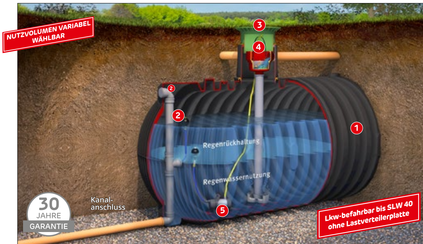
Abb. zeigt Carat XXL Retentionszisterne Plus mit Carat XL/XXL Retention Ausbaupaket 2 (Zubehör Seite. 155) und Technikpaket Garten-Komfort (Zubehör S. 66)
