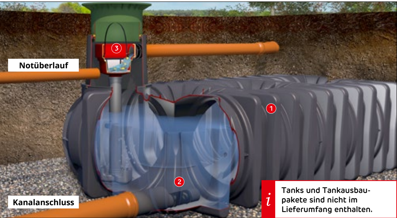
Abb. zeigt EcoFlow Control Ausbaupaket im Platin XL mit Platin Ausbaupaket
