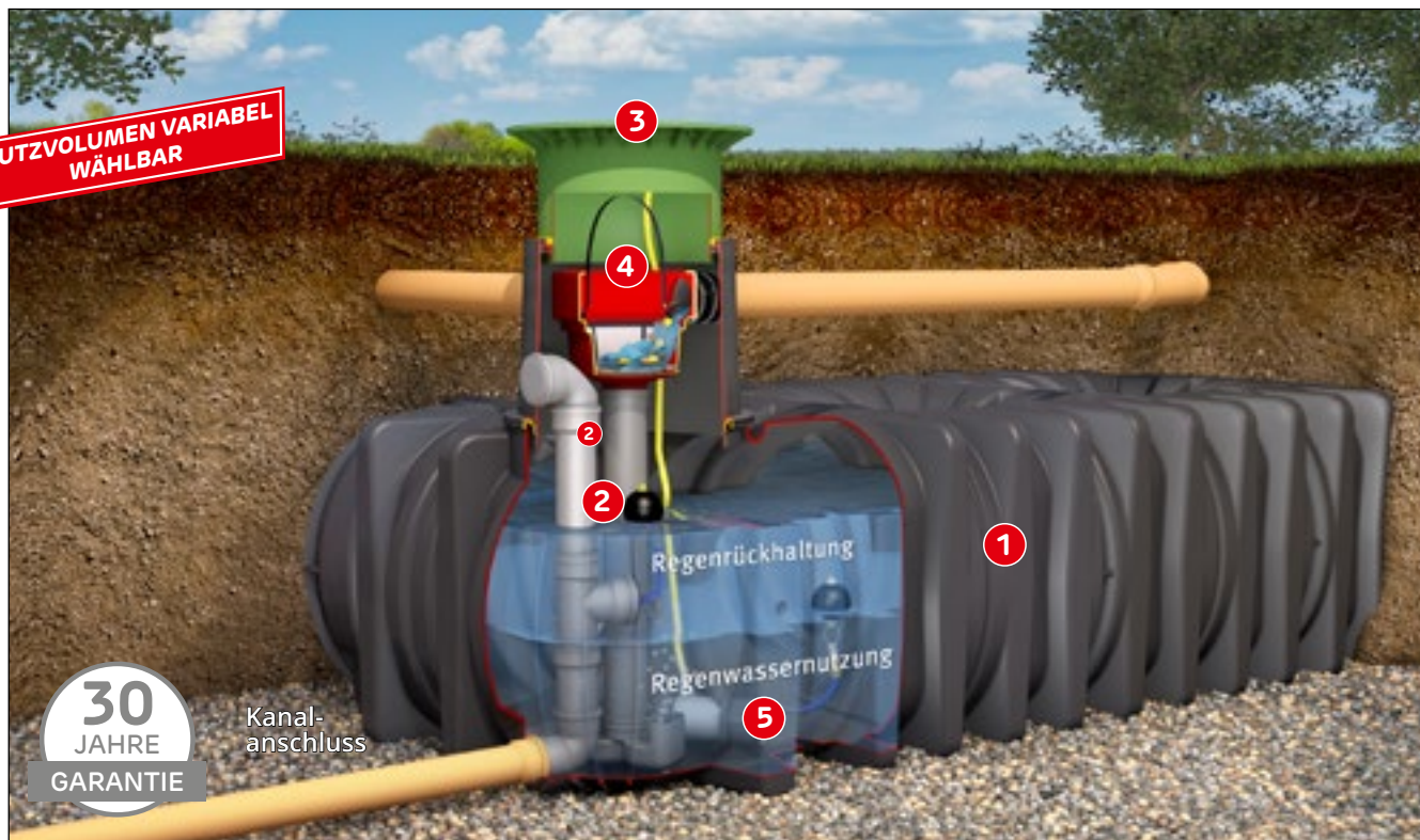
Abb. zeigt Platin XL Retentionszisterne mit Platin XL/XXL Retention Ausbaupaket 2 (Zubehör unten) und Technikpaket Garten-Komfort (Zubehör Seite 42)
