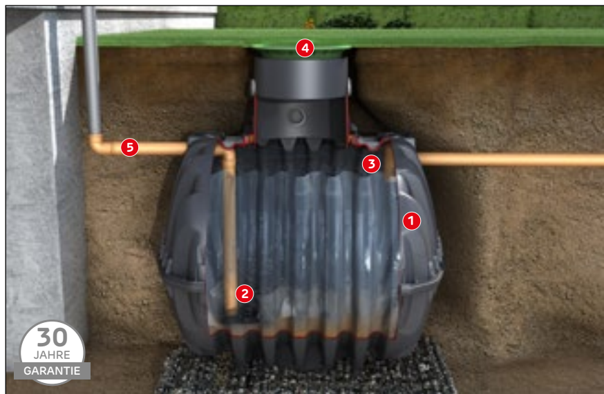
Abbildung zeigt Erdtank Carat M 153 Sedimentationstank mit Lieferumfang und Teleskop-Domschacht Mini (Zubehör S. 142)
