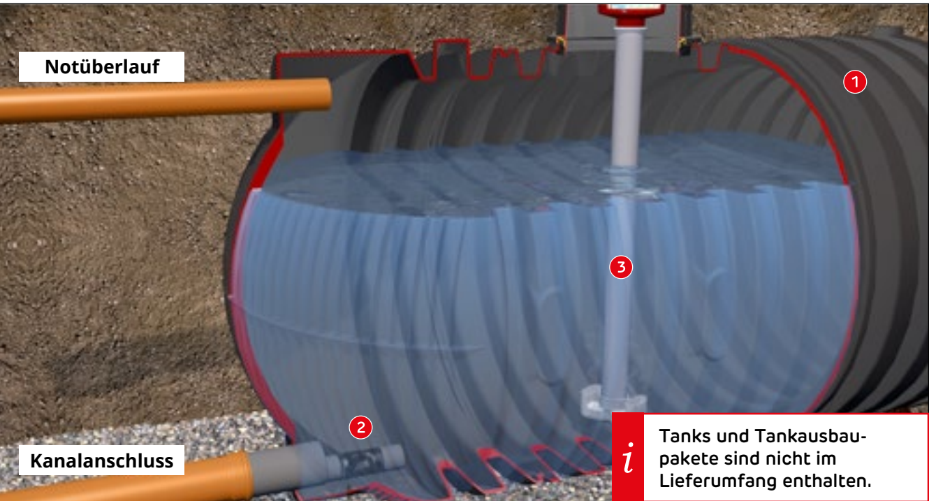
Abb. zeigt EcoFlow Control Ausbaupaket im Carat XL mit Carat Ausbaupaket
