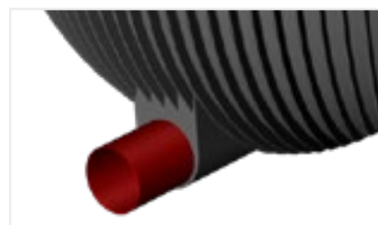
Verbindungsstutzen DA250 Zur Verbindung mehrerer Carat XXL Löschwassertanks (optional bis DA315)
