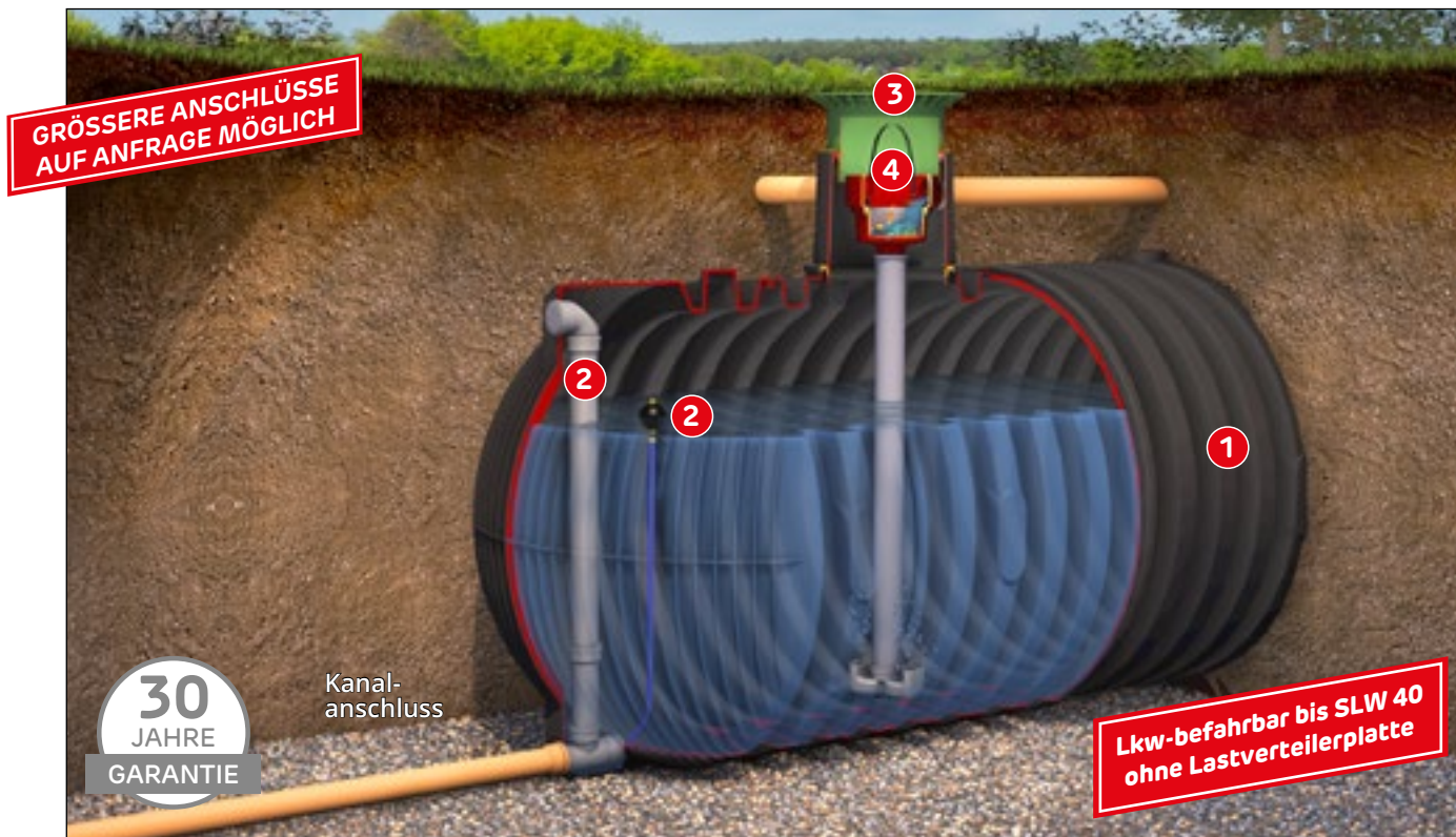
Abb. zeigt Carat XXL Retentionszisterne mit Carat XL/XXL Retention Ausbaupaket 2 (Zubehör S. 151)
