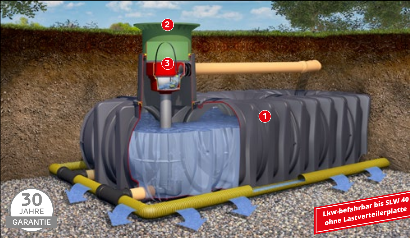
Abbildung zeigt Platin XL Versickerung mit Platin XL Retention/Versickerung Ausbaupaket 2 (siehe Zubehör S. 36)
