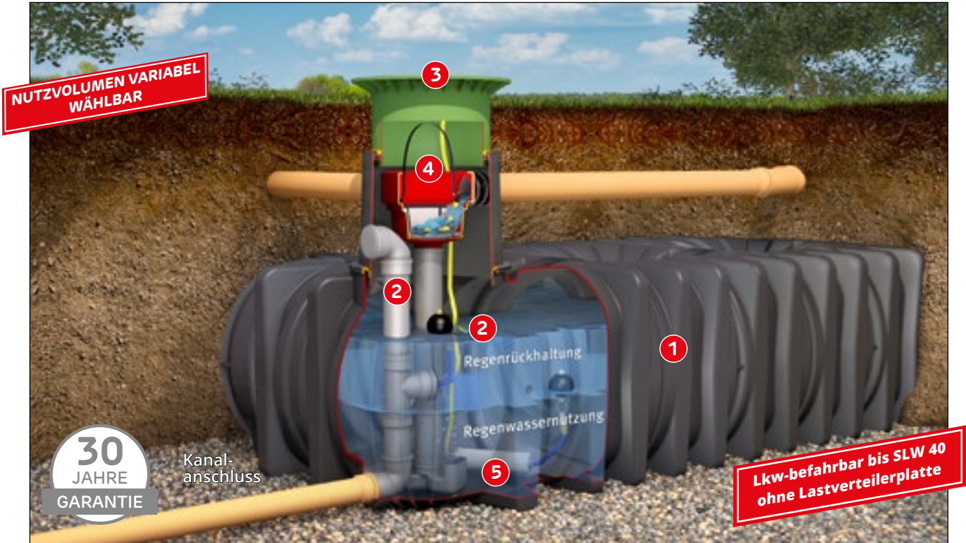
Abb. zeigt Platin XL Retentionszisterne mit Platin XL/XXL Retention Ausbaupaket 2 (Zubehör unten) und Technikpaket Garten-Komfort (Zubehör S. 38)
