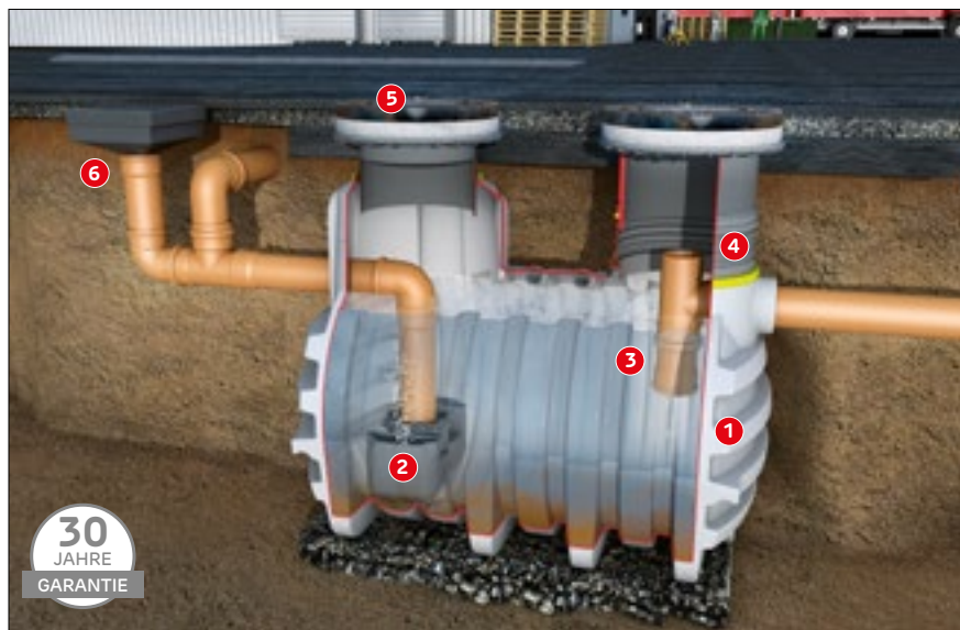
Abbildung zeigt Erdtank Diamant M 153 Sedimentationstank mit Lieferumfang und 2 x Teleskop-Domschacht, 2 x Betonabdeckung (Zubehör Seite 146) und Lastverteilerplatte.
