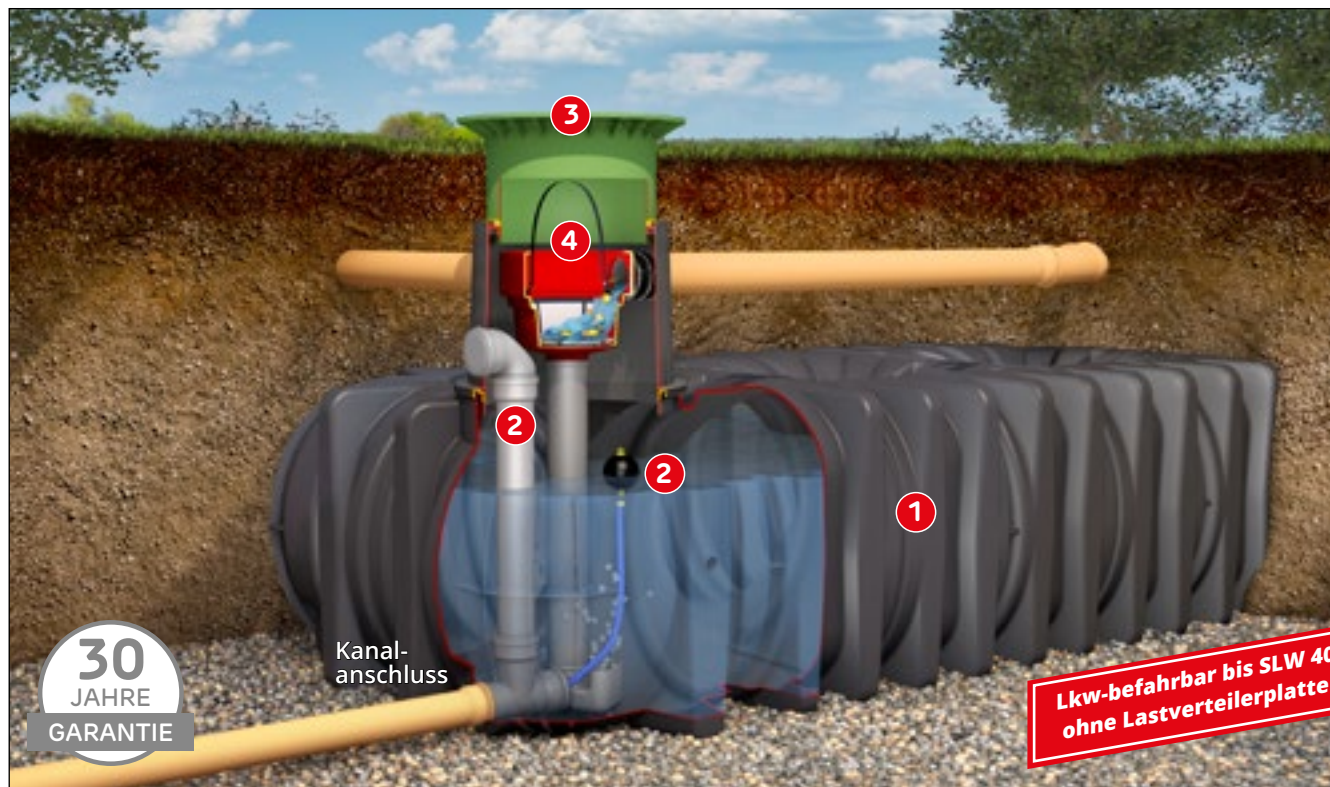
Abb. zeigt Platin XL Retentionszisterne mit Platin XL/XXL Retention Ausbaupaket 2 (Zubehör unten)
