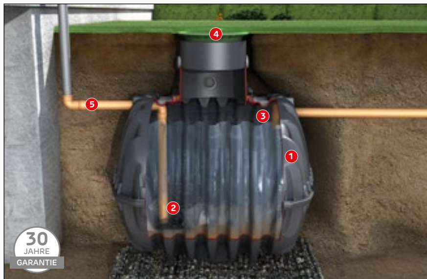
Abbildung zeigt Erdtank Carat M 153 Sedimentationstank mit Lieferumfang und Teleskop-Domschacht Mini (Zubehör S. 142)
