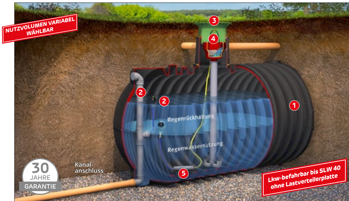
Abb. zeigt Carat XXL Retentionszisterne Plus mit Carat XL/XXL Retention Ausbaupaket 2 (Zubehör S. 151) und Technikpaket Garten-Komfort (Zubehör S. 62)
