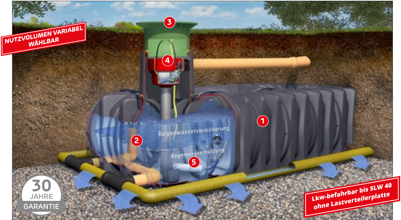
Abb. zeigt Platin XL Versickerung Plus mit Platin XL Retention/Versickerung Ausbaupaket 2 (siehe Zubehör) und Technikpaket Garten-Komfort (S. 36-38)
