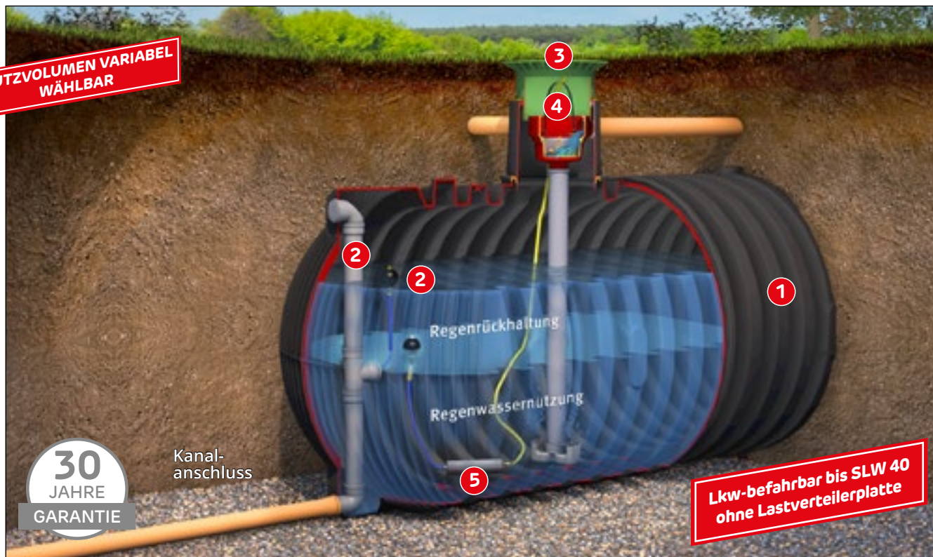
Abb. zeigt Carat XXL Retentionszisterne Plus mit Carat XL/XXL Retention Ausbaupaket 2 (Zubehör S. 151) und Technikpaket Garten-Komfort (Zubehör S. 62)
