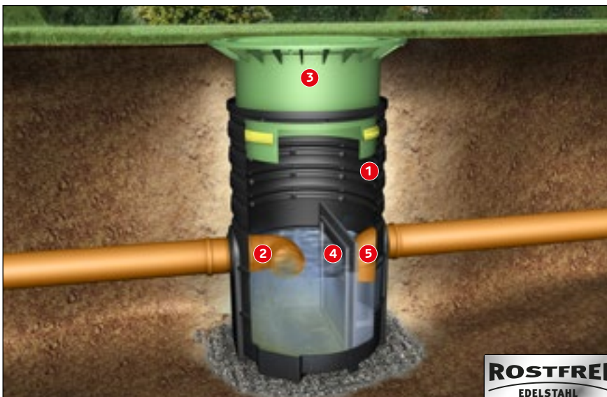
Abbildung zeigt SediProtect begehbar
